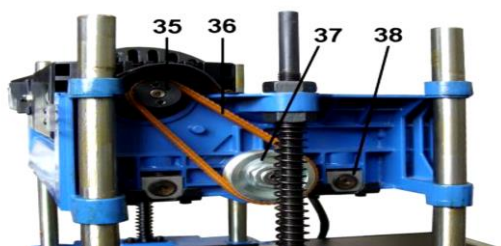
35 - ведущий шкив; 36 – ремень; 37 - ведомый шкив; 38 – подающий ролик
