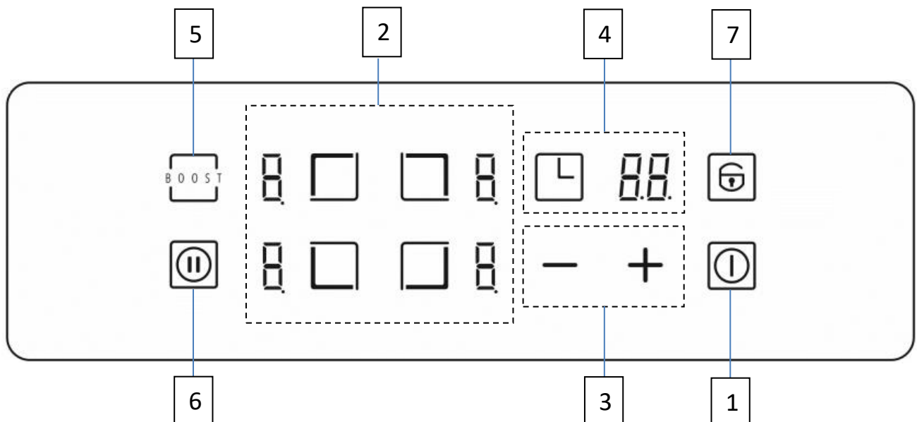
Рисунок 1 – Индукционная варочная панель ВНИ-6430А.ВК
